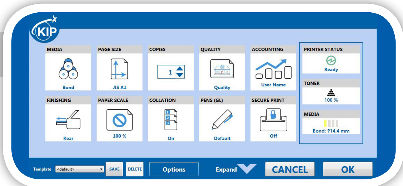
Windows® драйвер сжатый интерфейс
